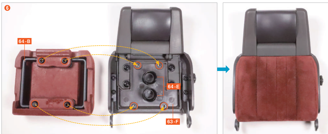
注意不要讓 64-E 脫落，將步驟 4 中組裝好的 64-B 的四個突起部分對準 63-F 上四個螺絲孔的凹槽，並嵌入固定。
